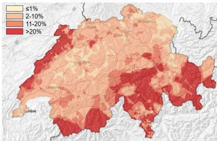
Radonkarte der Schweiz: Wahrscheinlichkeit den Referenzwert zu überschreiten Quelle: BAG, 2018
